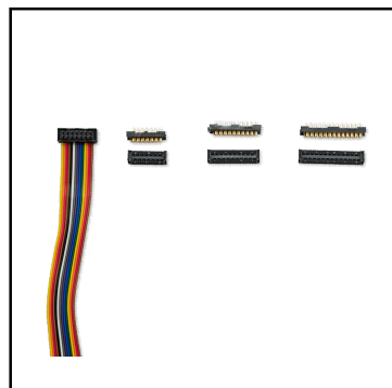
ヒロセHIF2E (HIF2E-14D-2.54RB)
