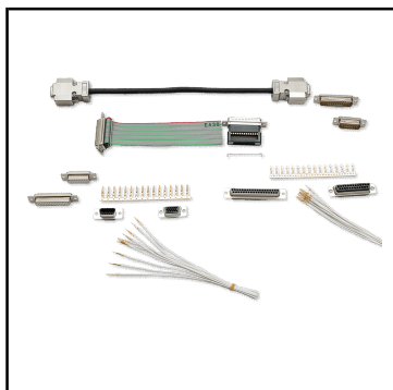
Dサブー覧 (圧着・半田・圧接)
