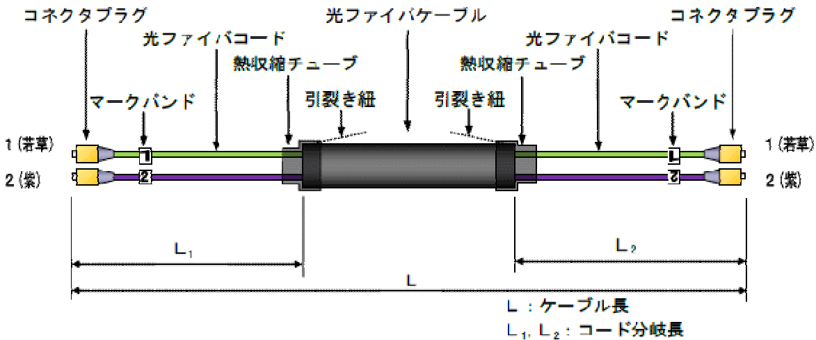
図3 両端コネクタ付の端末部の構成
